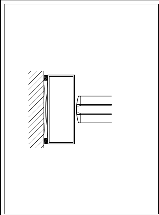
B DOOR SHOES / JAMB
