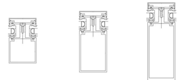
2-1/2" X 2-3/8"
